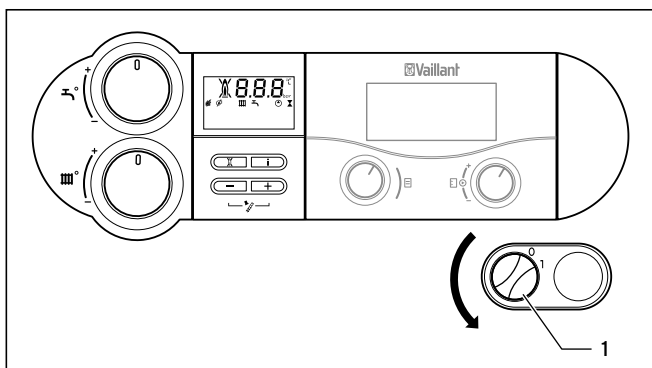
Рис. 4.13 Отключение прибора
